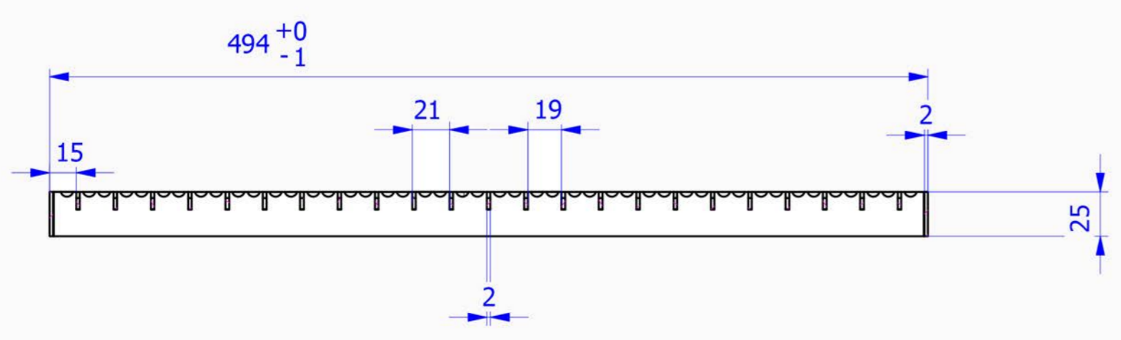
A-A ( 1 : 3 )
