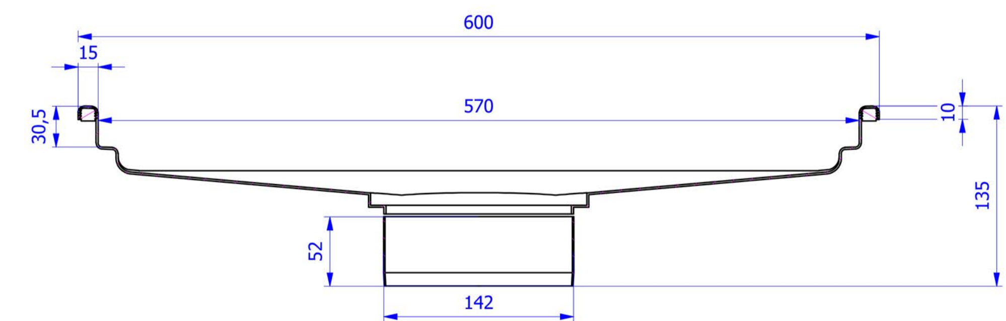
A-A ( 0,35 : 1 )
