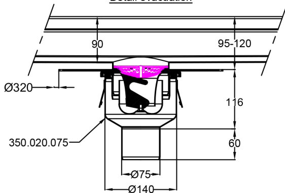
Détail évacuation
