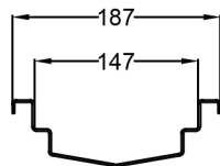
Profil caniveau
